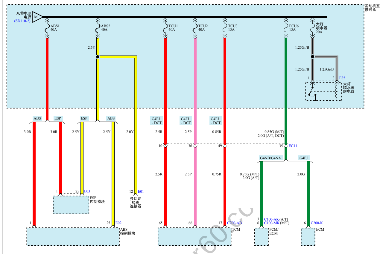
电源分布(3)
